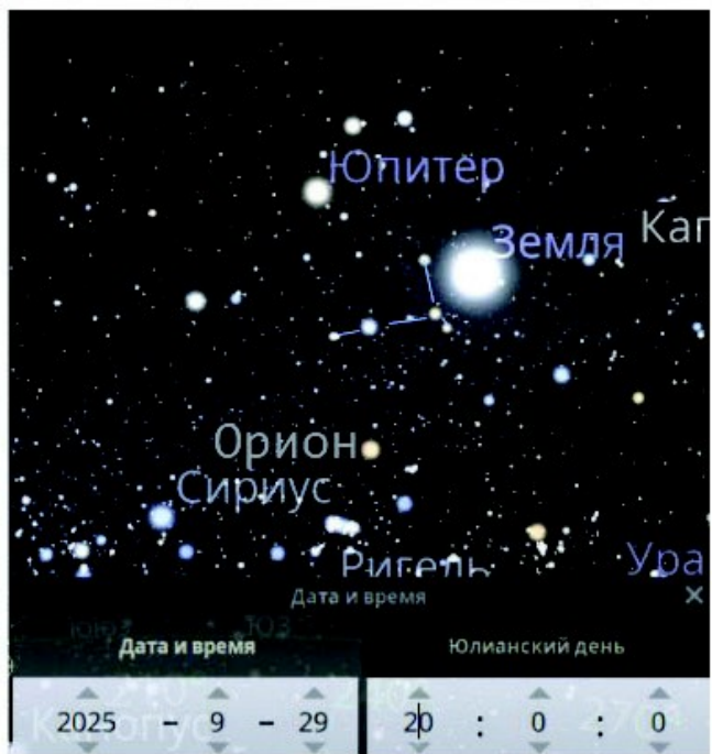
Рисунок 1-36. Смещение диска Земли на фоне звездного неба
