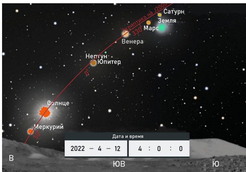
Рисунок 2-35. Звездное небо с Луны 12.04.2022 г. с эклипикой
