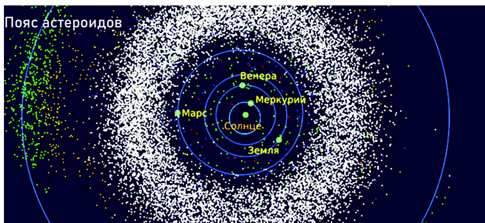
Рисунок 3-9. Схематическое расположение Марса и внутренних для Марса планет
