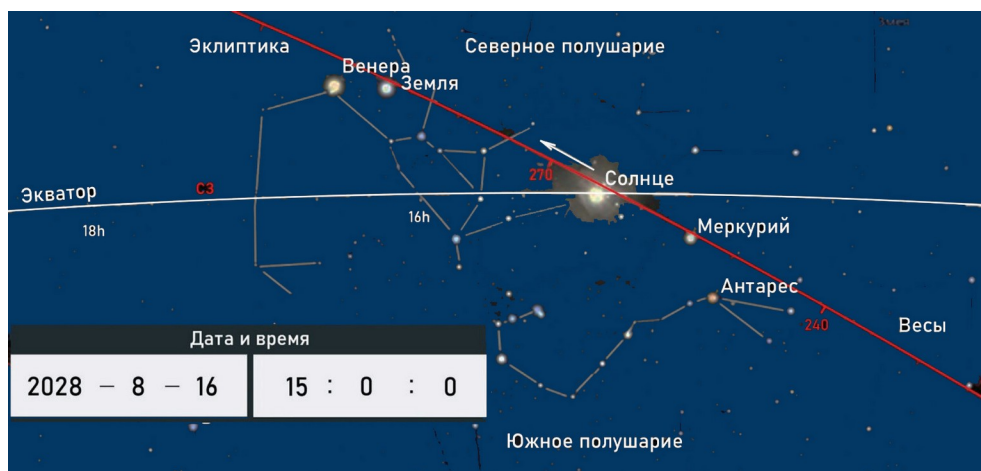
Рисунок 3-18. Точка весеннего равноденствия - точка пересечения экватора и эклиптики, через которую происходит переход Солнца из южного полушария в северное. Вид с Марса
